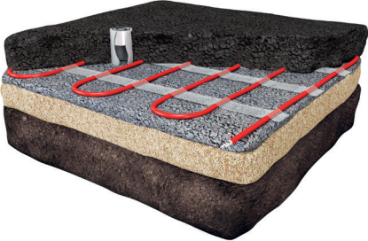
Manta Exterior Instalación en hormigón
