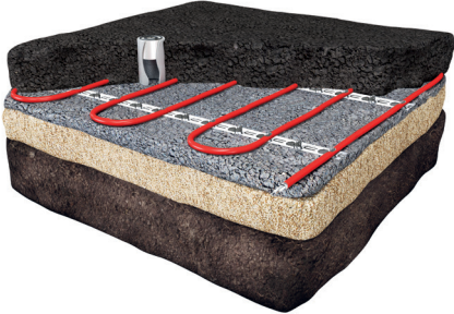
Cable Exterior Instalación en hormigón
