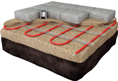
Manta Exterior Instalación bajo adoquines
